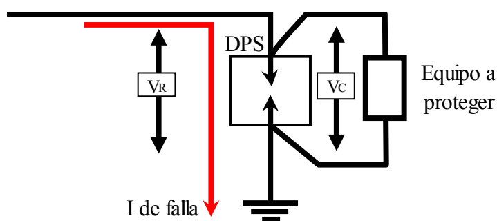
Figura 18. Montaje de los DPS
