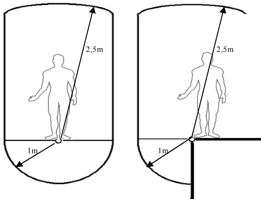
Figura 21. Distancias de seguridad contra contactos directos.
