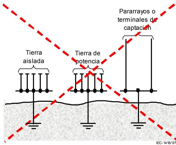
Figura 12. Puestas a tierra separadas o independientes (prohibido).
