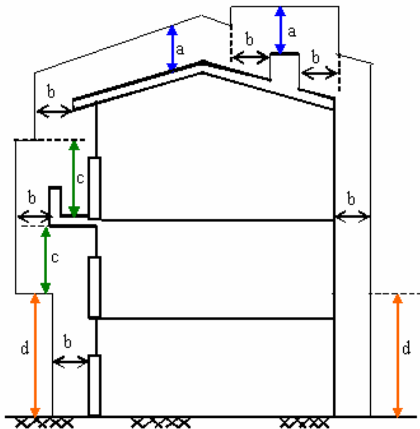
Figura 5. Distancias de seguridad en zonas con construcciones
