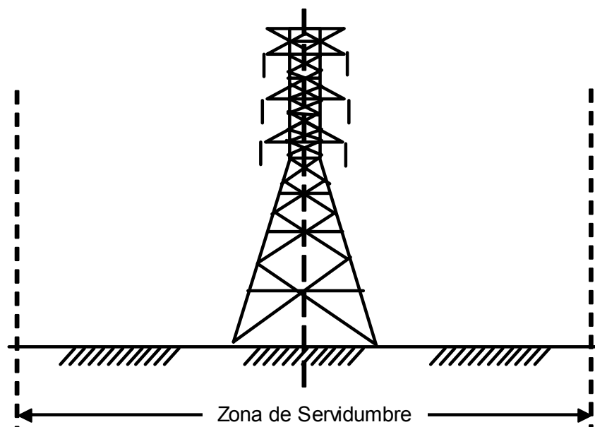
Figura 19. Ancho de la zona de servidumbre.
