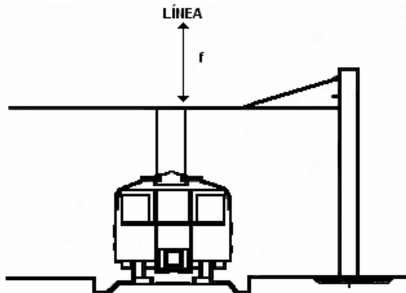
Figura 8. Distancia "f" en cruces con ferrocarriles electrificados.
